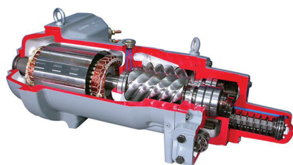
Compressoren
