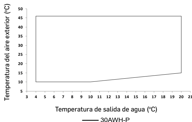
Rango de operación, modo refrigeración
