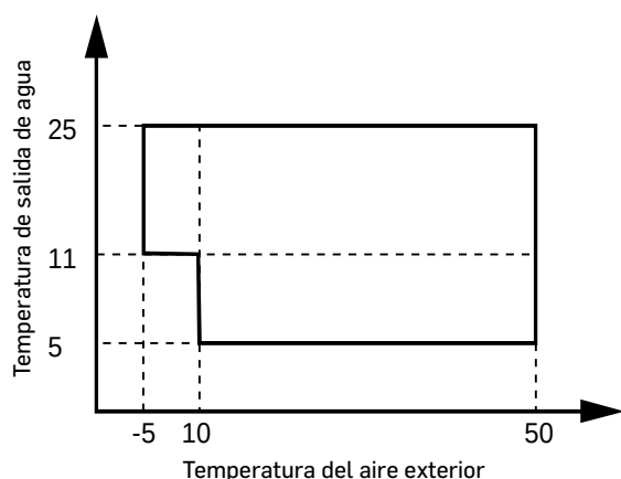
Rango de operación, modo refrigeración
