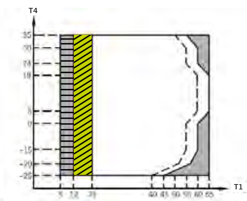
Operación en refrigeración
