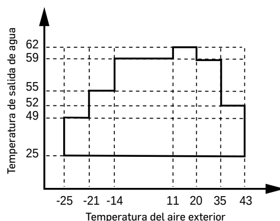
Rango de operación, modo calefacción
