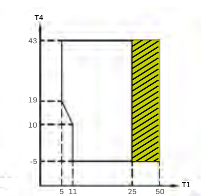
Operación en calefacción
